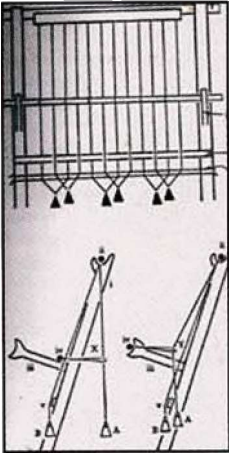
Şekil 4: "Çözgü ağırlıklı tezgâhın şematik çizimi (i)=Düz direkler (ii)=Kumaş levendi (iii)=Gücü sopası desteği (iv)=Gücü sopası. (v)=Ağızlık sopası (vi)=İpe aralıkları X doğal ağızlık; Y yapay ağızlık göstermektedir
