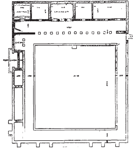
Abb. 271. Grundriss des unteren Gymnasiums.
